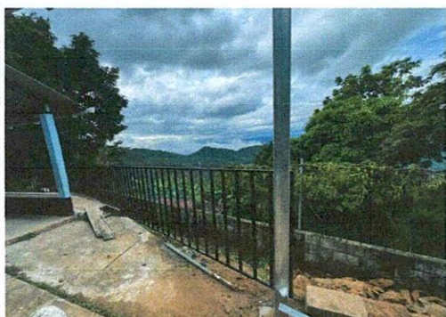
Foto 3: mejoramiento del cerco perimetral colocando baranda metalica para resguardar la integridad fisica de los niños y niñas de la etapa 4.
